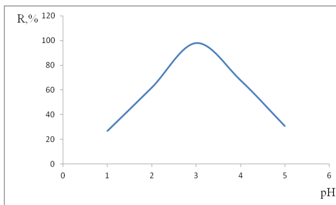
Рис.9. Зависимость степени сорбции висмута на модифицированном сорбенте от pH ( m_c=0,03 г; V_k=25 мл; C_{Bi^{3+}}=1 мг/л).
