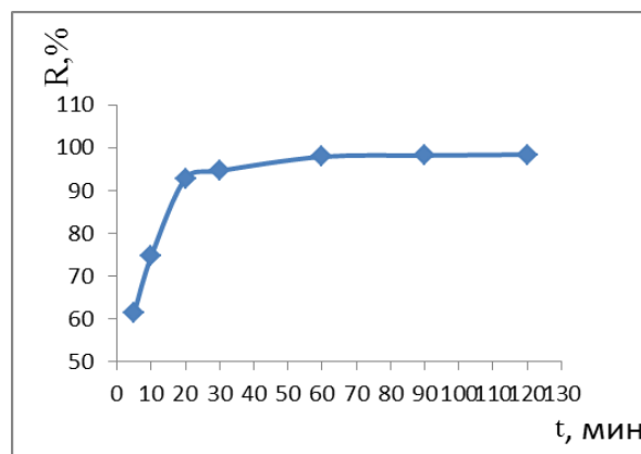
Рис.10. Зависимость сорбции висмута на модифицированном сорбенте от времени контакта фаз ( m_c=0,03 г; V_k=25 мл; C_{Bi^{3+}}=1 мг/л).
