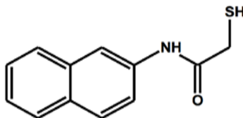
Рис.1. Структурная формула тионалида
