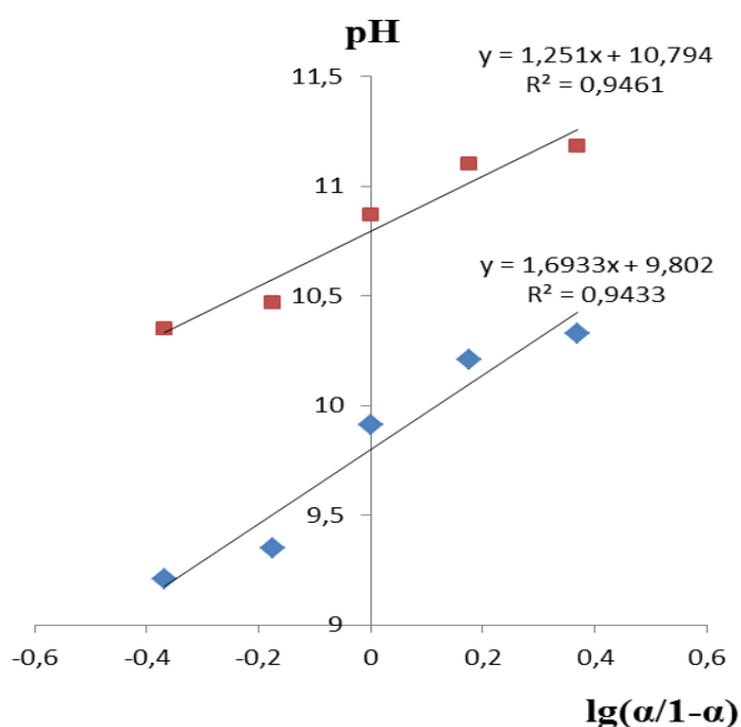
Рис. 2. Графическое определение констант ионизации ПАФАР
