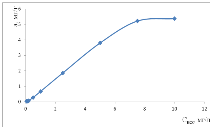
Рис.11. Кривая насыщения модифицированного сорбента АВ-17-Гл висмутом ( m_c=0,03\text{г} ; \text{pH } 3,0 ; C_{исх} = 0,05 \div 10 \text{ мг/л} )
