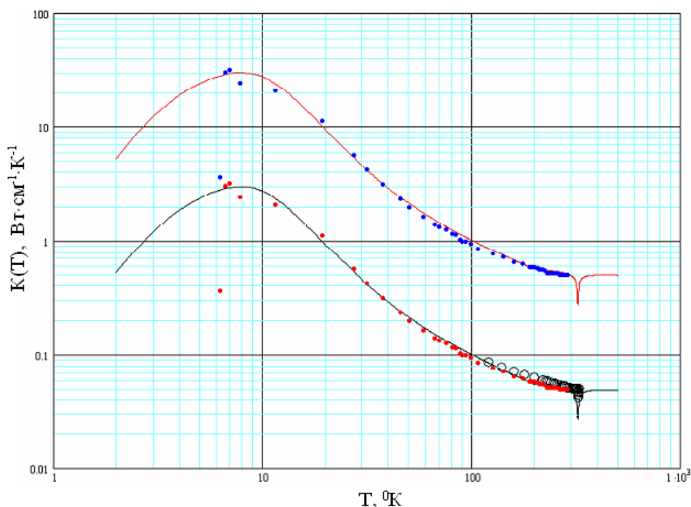
Рисунок 1. Температурная зависимость теплопроводности «номинально чистых» кристаллов ТГС в широком интервале температур 6-340^{\circ}K [1-3]. Сплошные линии – расчет; нижняя кривая K(T) смещена вниз на порядок и при T > 100^{\circ}K кружочками приведены данные из [3].
